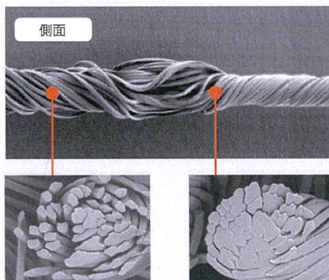
断面1
